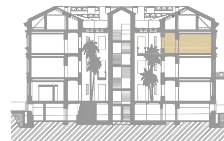
Byt B3.02 - vyznačen v řezu
