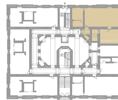
Byt B1.02 - vyznačen v půdorysu 1.NP
