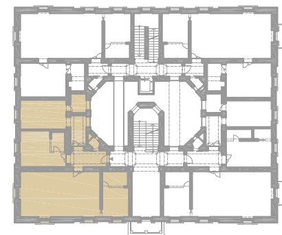
Byt A2.04 - vyznačen v půdorysu 2.NP
